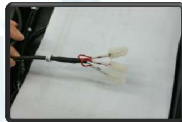
Robot Cable
